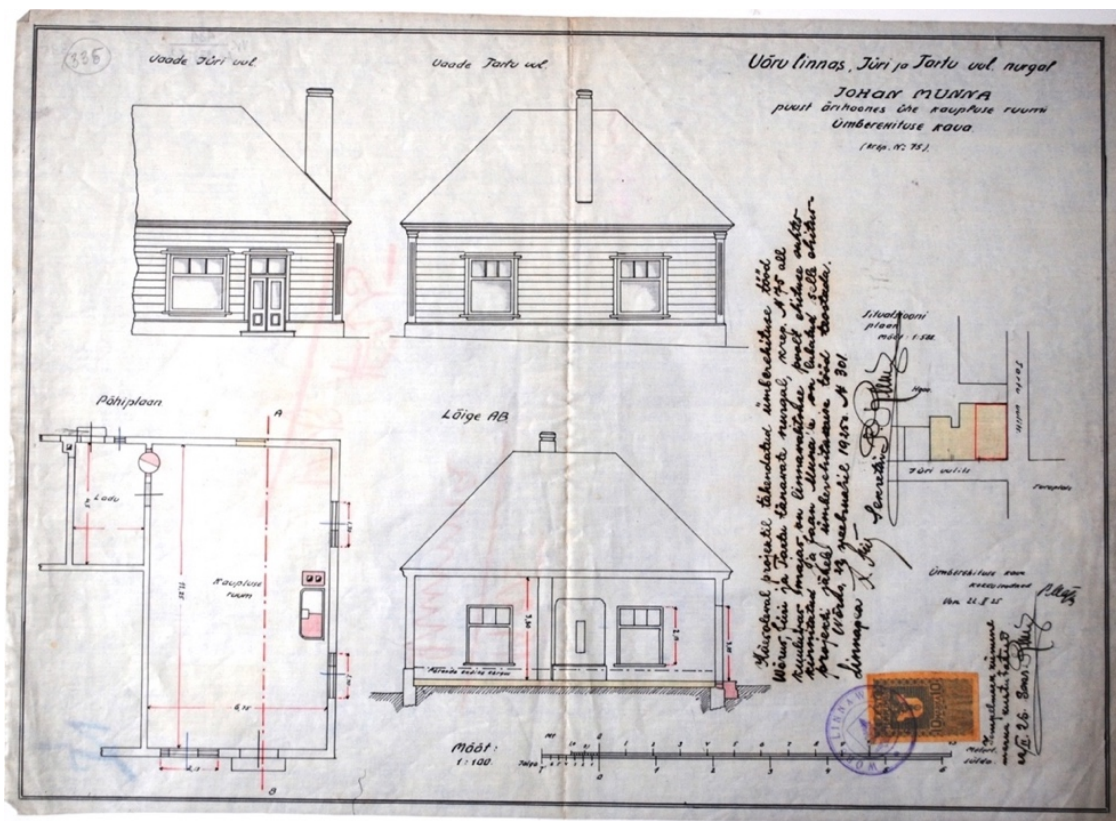
Kaupluse ühe ruumi ümberhitamise plaan. Jüri tn ja Tartu tn nurgal. Ehitaja Johan Munna. joonis: Võrumaa Muuseum, VK _ 484:63 Ar 279:63
